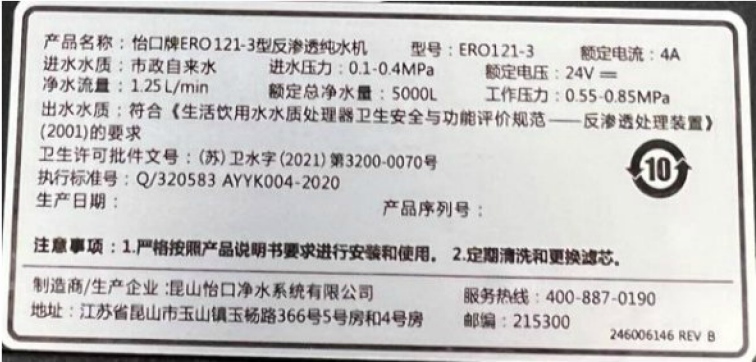
ERO121-3（铭牌）
